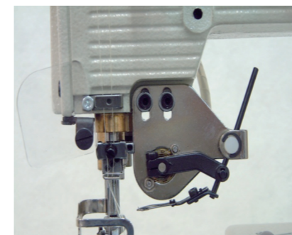
■ EW 電気式上糸払い (電気式ワイパー WX, RX, NM 用) ELECTRIC TYPE WIPER FOR WX, RX, NM DESILIZADOR ELECTRICO PARA WX, RX, NM 电动式上勾线
