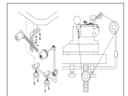
■ RT-1 ゴム張り装置 (手動式) RX-PHK Elastic expander device ( manual operation ) RX-PHK EXPANDIDOR DE ELASTICO RX-PHK 松紧带撑开装置
