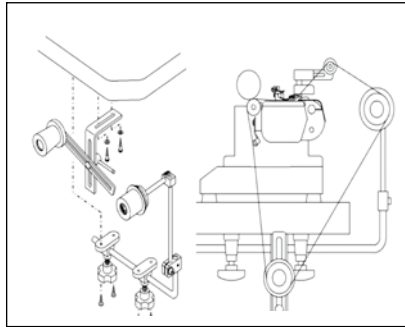
■ RT-2 ゴム張り装置 (手動式)NR-PHK Elastic expander (Manual operation) NR-PHK EXPANDIDOR DE ELASTICO NR-PHK 松紧带撑开装置
