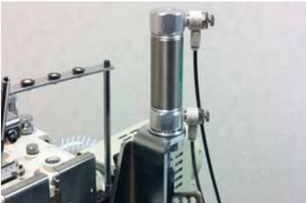
■ FL エアー式押え上装置 AIR TYPE FOOT LIFTER LEVANTA PIE NEUMATICO 气压式抬压脚装置
