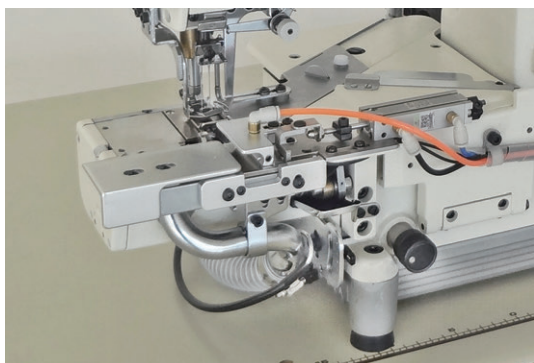
■ ABH-1A 裾巻き縫い開閉フォルダ装置（センサー式） for NR,NRE,NC Sensor type pneumatic hemming guide for NR, NRE, NC
