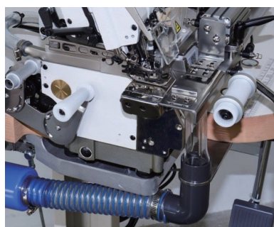
■ RT-4 ゴム張り装置（固定式） for JJ Fixed type expansion roller for JJ
