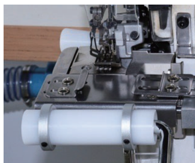
■ RT-4-AF ゴム張り装置（エア開閉式） for JJ カフ部分やネックリブ付に Pneumatic expansion roller for JJ for cuffs and neck ribs
