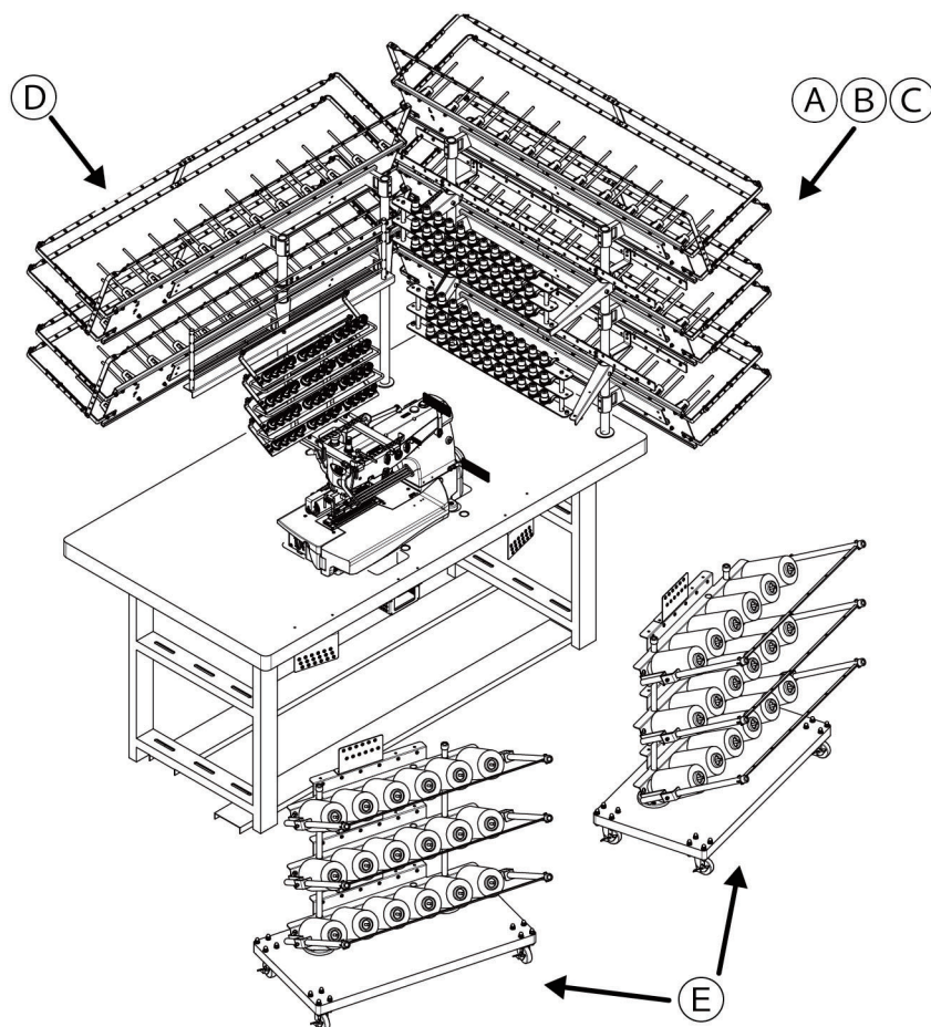
② 下糸ゴム用 (ET) for lower thread(ET)
