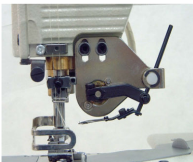
■ EW 電気式上糸払い装置 (電気式ワイパー Nfor W,NR,NC) Electric type wiper for NW, NR, NC
