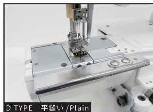
D TYPE 平縫い / Plain
