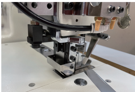
■ TC1・2 テープカッター（エアー式） for NL,SQ Air type tape cutter for NL, SQ
