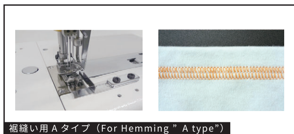
裾縫い用 A タイプ (For Hemming " A type")
