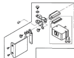
■ LED LED ライト LED right 各モデルに装着可能です。 It can be installed on each model.
