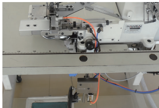
■ ABH-1M 裾巻き縫い開閉フォルダ装置（手動式） for NR,NRE,NC Pneumatic hemming guide with knee switch for NR, NRE, NC
