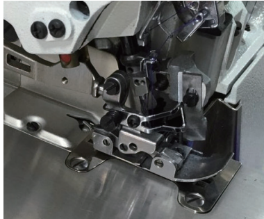
■ HTC 横型空環切り装置 for JJ Horizontal chain cutter for JJ
