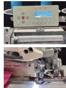
■ ATC 自動テープカット装置（センサー式） for JJ 自動、半自動で縫製前後の糸生地始末（カット）を行います。 Auto tape cutting device Automatically or semi-automatically cuts the thread fabric before and after sewing.
