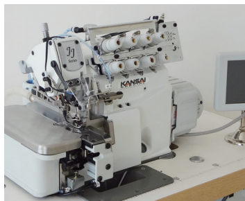
■ BL 自動バックラッチ装置（センサー式） for JJ 空環を縫い目に巻き込み、始末の手間を軽減。 Auto backlatch device for JJ The chain is wrapped around the seam to reduce the effort required for cleaning.
