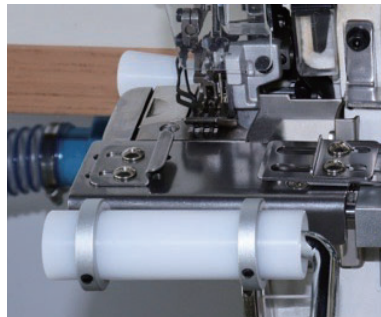
■ RT-4-AF ゴム張り装置（エアー開閉式） for JJ カフ部分やネックリブ付に Pneumatic expansion roller for JJ for cuffs and neck ribs
