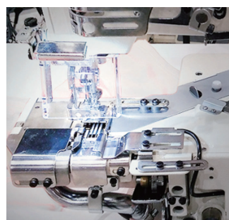
■ LED LED ライト LED right 各モデルに装着可能です。 It can be installed on each model.
